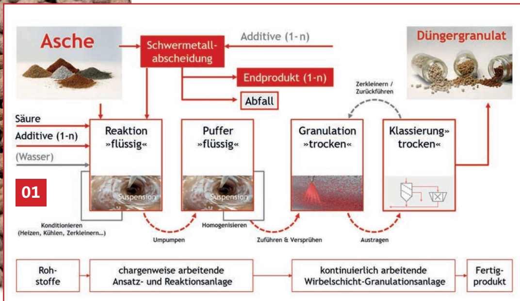
01 Das zweistufige Verfahren gliedert sich in den Aufschluss des in der Asche eingebundenen Phosphors und einen Sprühgranulationsprozess, der zu direkt marktfähigen Endprodukten führt
